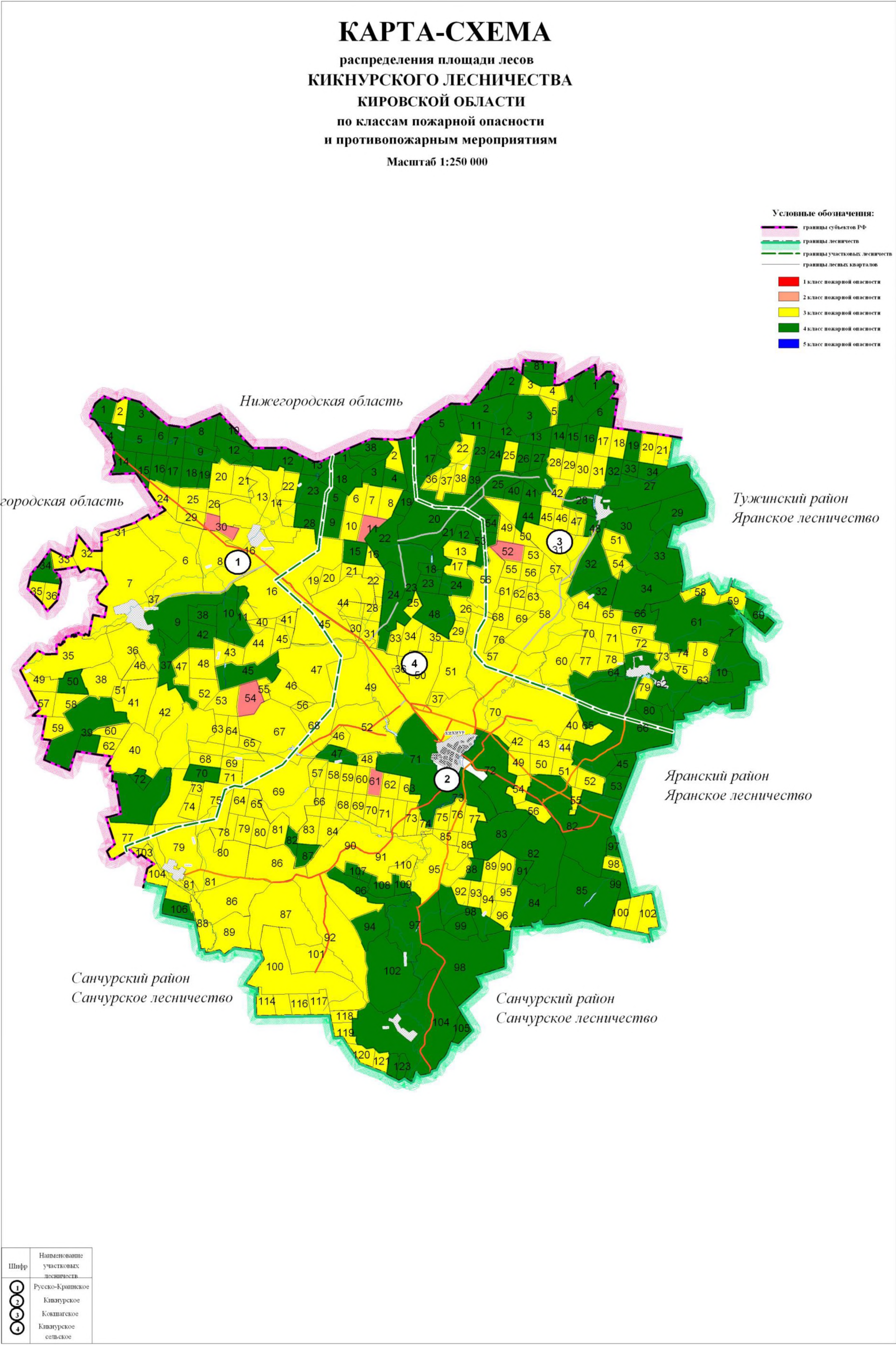
Рисунок 5. Карта-схема распределения площади лесов Кикнурского лесничества Кировской области по классам пожарной опасности и противопожарным мероприятиям
